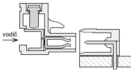
Svorkovnice - zásuvka pro zasunutí do vidlice na tištěném spoji, montáž vodiče pod šroub (u některých typů pod pružnou lamelou)
