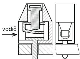
Montáž vodiče pod šroub s ochranou vodiče pružnou lamelou
