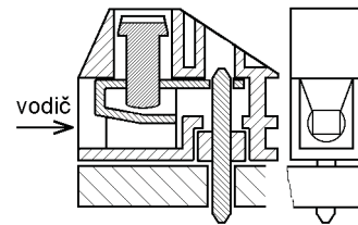
Svorkovnice nasouvací na kolíkovou lištu, montáž vodiče pod šroub
