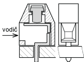
Montáž vodiče pod šroub s ochranou vodiče pružnou klecí
