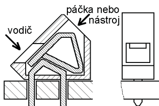
Bezšroubová montáž vodiče s pomocí nástroje nebo páčky, která je součástí svorkovnice
