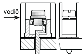
Svorkovnice s přepážkami s montáží do do ploš. spoje
